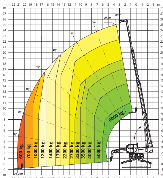
ARGANO 3.500 kg
